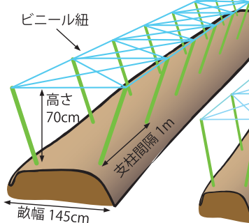
図3 誘引用の平棚
